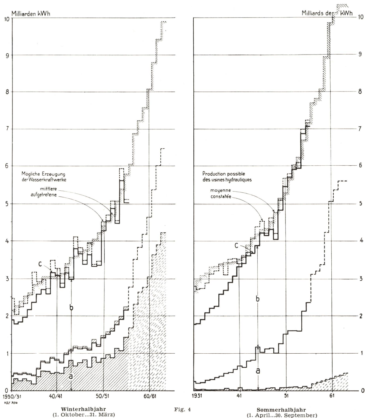
Technisch mögliche und wirkliche Energieerzeugung der Wasserkraftwerke der Allgemeinversorgung Die Kurven rechts der Ordinate 1955/56 zeigen die voraussichtliche Zunahme der mittleren Produktionsmöglichkeit durch die Fertigstellung der in Abschnitt I, Ziffer 3, abzüglich der in Abschnitt II, Ziffer 4, erwähnten Kraftwerke. a Erzeugung in Speicherwerken, wovon schraffierter Teil aus Saison-Speicherwasser b Erzeugung in Laufwerken, wovon schraffierter Teil aus Saison-Speicherwasser c Gesamte Erzeugung in Wasserkraftwerken
