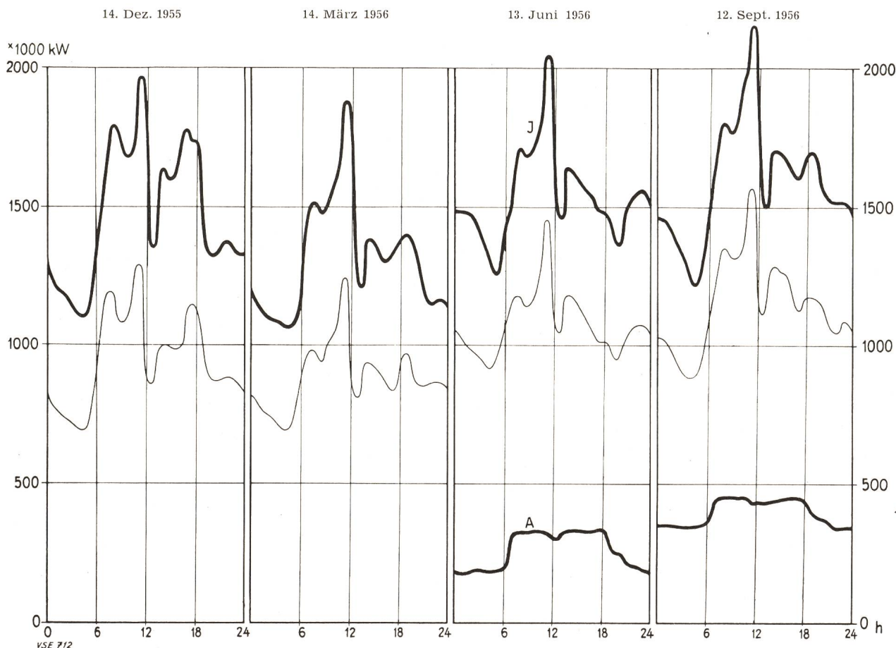
Fig. 9 Verlauf des Inlandverbrauches und des Ausfuhrüberschusses an Mittwochen J Inlandverbrauch, dünn gezeichnete Kurve Inlandverbrauch 1949/50 A Ausfuhrüberschuss
