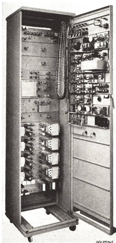
Fig. 10 Recheneinheit des Pile-Simulators mit geöffneter Türe
