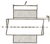
Fig. 3 Spaltlänge l und Durchmesserunterschied u bei umlaufenden Wellen
