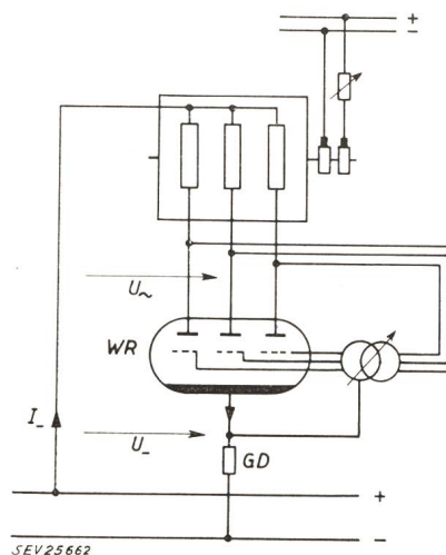
Fig. 4 Prinzipschaltung eines Stromrichtermotors I_- Gleichstrom; U_- Gleichspannung; U_{\sim} Wechselspannung; GD Glättungsdröhselspule; WR Wechselrichter
