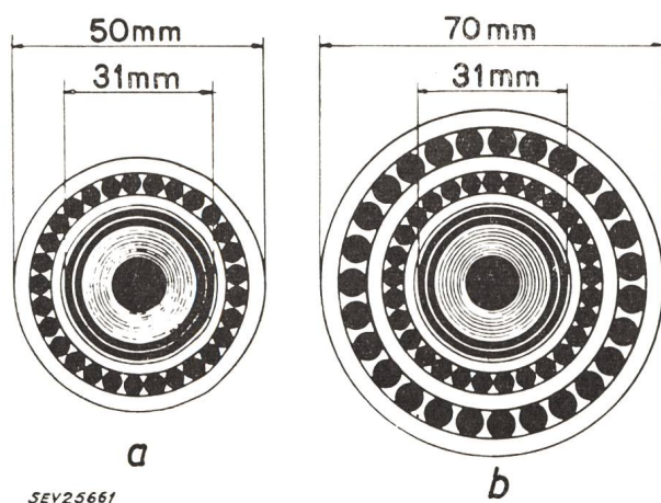
Fig. 3 Aufbau des Gleichstrom-Hochspannungskabels der Gotlandübertragung a Seekabel; b Kabel in Küstenähe
