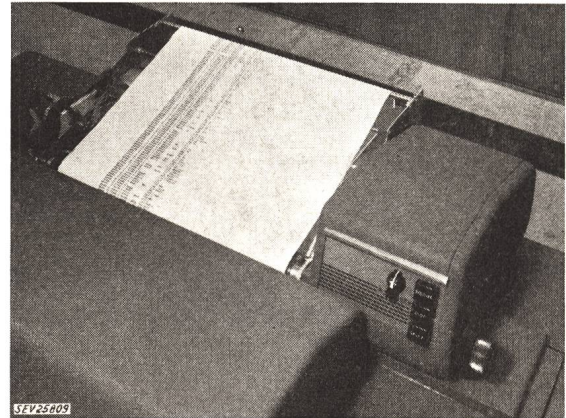
Fig. 9 Druckwerk
