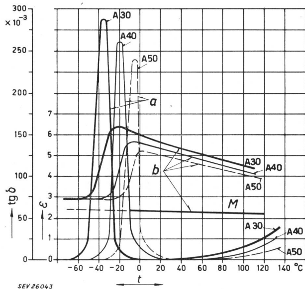
Fig. 1 Verlustfaktor (a) und Dielektrizitätskonstante (b) verschiedener Imprägnierungsmittel in Funktion der Temperatur t Temperatur; \text{tg}\delta Verlustfaktor; \epsilon Dielektrizitätskonstante; A30, A40, A50 Typenbezeichnungen für Clophenes; M Mineralöl
