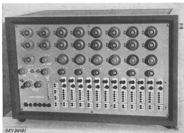
Fig. 2 Klein-Analogierechengerät
