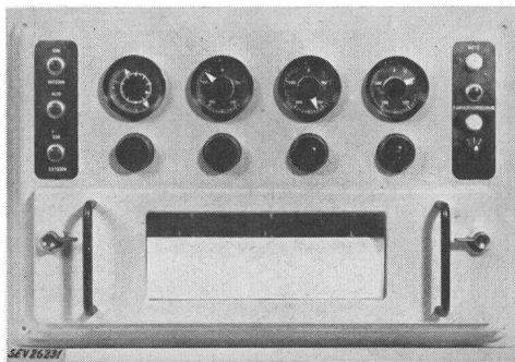
Fig. 8 Dreifach-Servoschreiber
