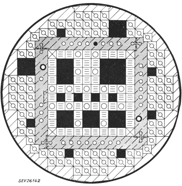
Fig. 1 Schematischer Plan des ETR-Reaktors (Durchmesser 80,6 cm) Legend: ⊗ Wasser-Aluminium-Reflektor; ○ Regelelemente; ≡ Füllelemente; □ Kontrollstäbe; ■ Experimentierraum; ▨ Beryllium-Reflektor; ◊ Al-Reflektor; ● Quelle; ○ zurückziehbare Elemente für weitere Experimente
