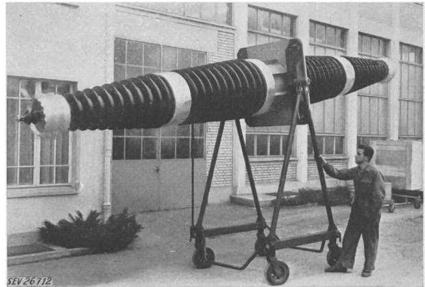
Fig. 1 Freiluft-Mauer-Durchführung für 660 kV Prüffeldbetrieb Typ CMffh 660 Pm
