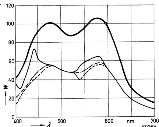
Fig. 3 Darstellung des Spektrums einer «Daylight»-Lampe \lambda Wellenlänge; W relative spektrale Energieverteilung — nicht kompensiert — — — kompensiert — · — · korrigiert
