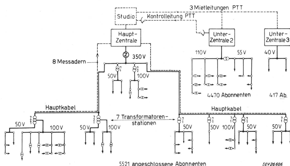
Fig. 5 Prinzipschema des Betriebes der Radibus Basel A.-G.
