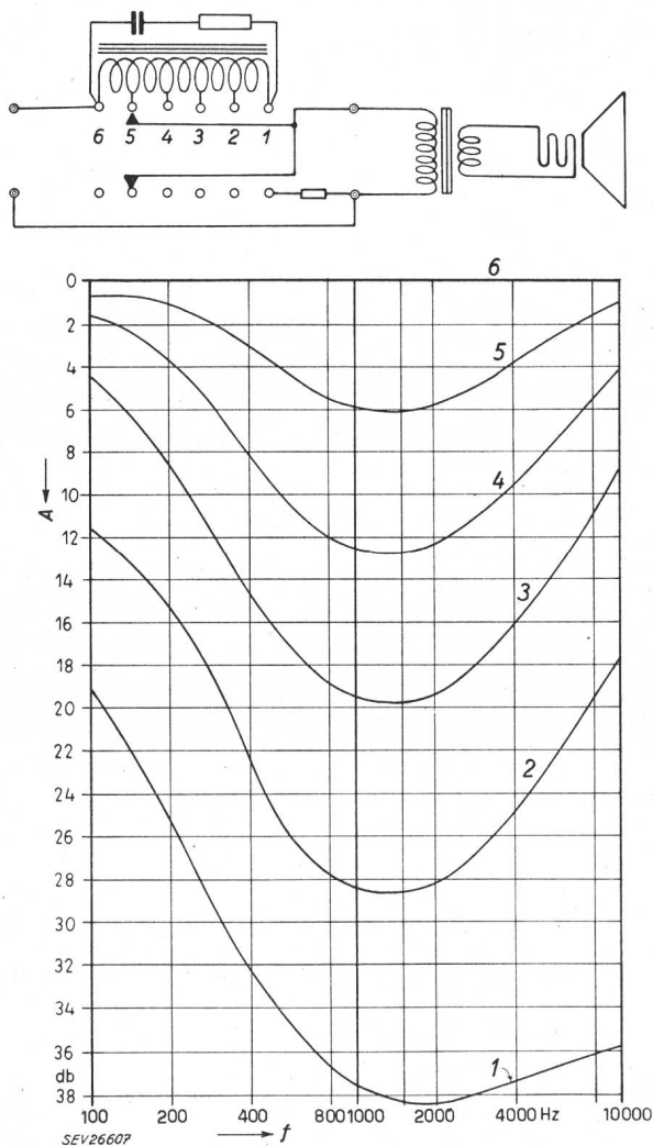
Fig. 6 Schaltschema und Charakteristiken 1...6 des physiologischen Lautstärkeregers A Abschwächung; f Frequenz
