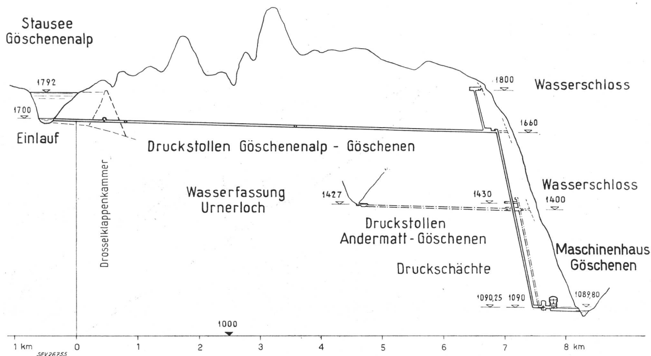
Fig. 5 Längenprofile
