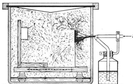
Fig. 2 Geschlossener Kasten und Zerstäuber für die Prüfung der Feuchtigkeitsbeständigkeit 1 Prüfling 2 Pressluft
