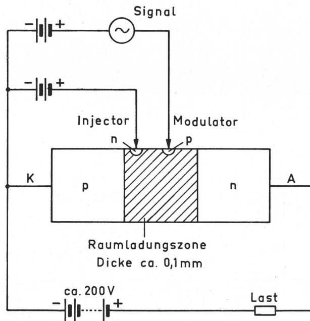
Fig. 17 Prinzipieller Aufbau der Spacistor-Tetrode
