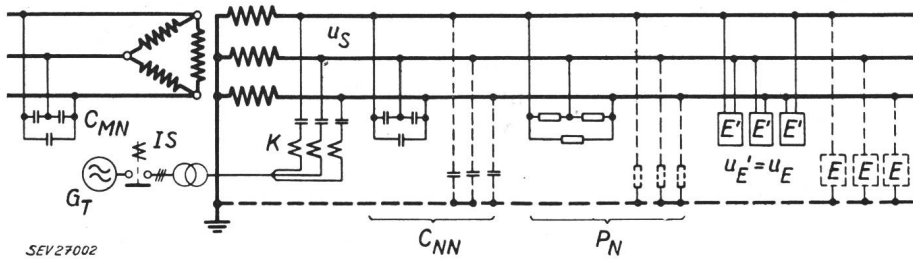
Fig. 2 Parallelankopplung dreiphasiger Signalströme an das Niederspannungsnetz (Wenn kein Nulleiter vorhanden ist, fallen die gestrichelt gezeichneten Partien weg) G_T Tonfrequenzgenerator; IS Impulsschütz; K Kopplungsmittel; E Empfangsgeräte, Anschluss Phase/Null; E' Empfangsgeräte, Anschluss Phase/Phase; P_N Netzbelastung (Wirkkomponente); C_{NN} Kondensatoren im Niederspannungsnetz; C_{MN} Kondensatoren im Mittelspannungsnetz; u_s relative Sendespannung; u_E relative Empfangsspannung Phase/Null; u_{E'} relative Empfangsspannung Phase/Phase; u_s, u_E, u_{E'} pro Volt der Netzspannung
