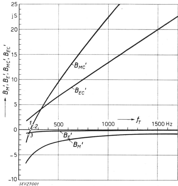
Fig. 1 Blindleitwerte in jS pro 0,144 MW Wirkbelastung in Funktion der Tonfrequenz f_T , bezogen auf 0,38 kV B_M' = 23,3 \frac{f_N}{f_T} Blindleitwert von unkompensierten Motoren B_E' = 2,3 \frac{f_N}{f_T} Blindleitwert von unkompensierten Entladungslampen und Schweissapparaten B_{MC}' = 1,17 \frac{f_T}{f_N} - 23,3 \frac{f_N}{f_T} Blindleitwert von kompensierten Motoren B_{EC}' = 0,67 \frac{f_T}{f_N} - 2,3 \frac{f_N}{f_T} Blindleitwert von parallelkompensierten Entladungslampen und Schweissapparaten f_N Netzfrequenz Punkt 1 liegt bei +j1S, 240 Hz, Punkt 2 bei 0S, 223 Hz und Punkt 3 bei -j1S, 200 Hz
