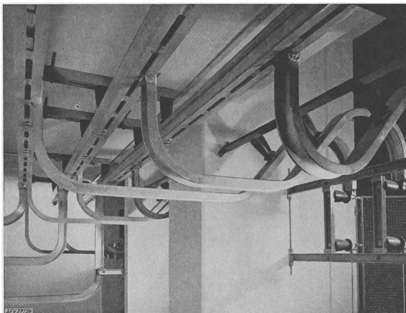
Fig. 4 Abzweigung von den Sammelschienen mit Einfach-U-Profil
