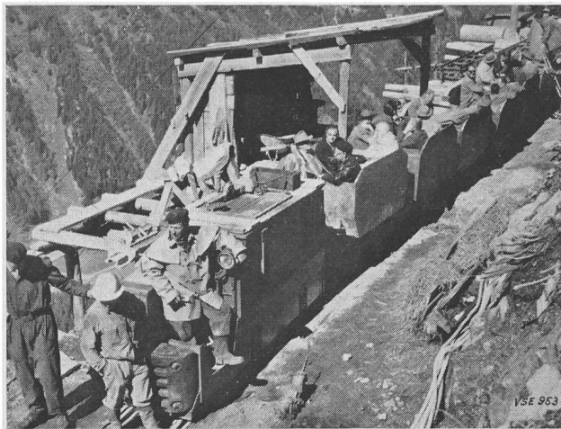
Fig. 2 Stollenbahn Murtaira—Plancanin
