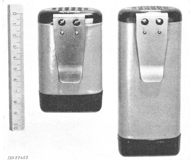
Fig. 9 Rufempfänger RE16
