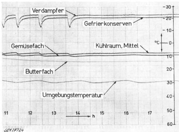
Fig. 2 Temperatur-Registrierstreifen eines Kühlschranks, aufgenommen mit dem Sechsfarbenschreiber
