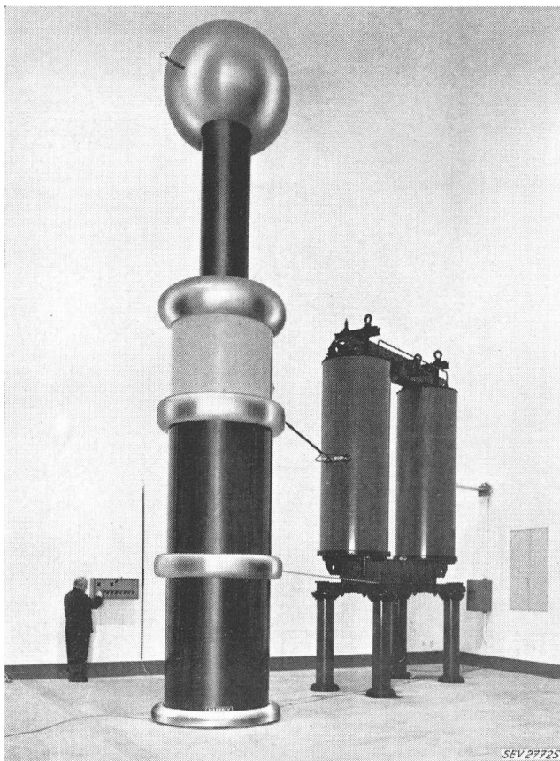
Fig. 3 Transformator-Kaskade für Spannungen bis 1000 kV, 50 Hz
