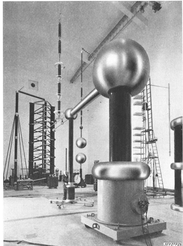
Fig. 4 Radiostörspannungs-Messplatz für Hochspannungsmaterial bis max. 420 kV Betriebsspannung
