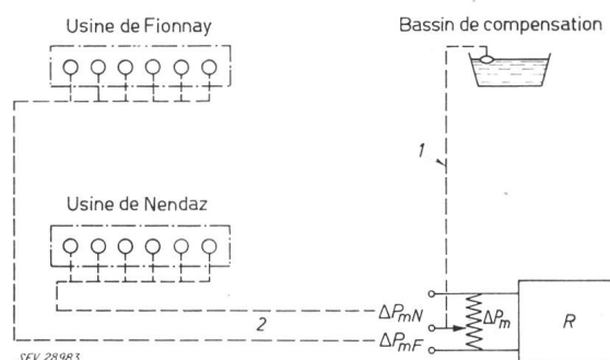
Fig. 6 Répartition des ordres de réglage \Delta P_m sur les 2 usines de Fionnay-Dixence et de Nendaz par le Régulateur de réseau R 1 télécommande; 2 ordres de réglage Signification des symboles voir légende à la fig. 4
