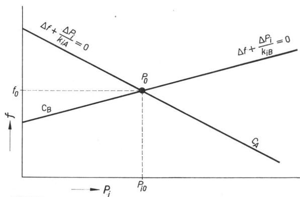
Fig. 3 Caractéristique du réglage fréquence-puissance de deux réseaux interconnectés
