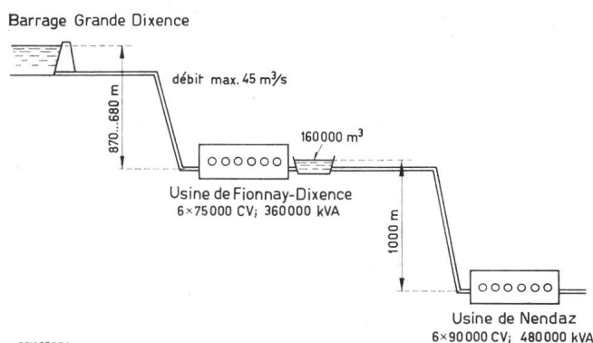
Fig. 4 Disposition des 2 usines de Fionnay et de Nendaz
