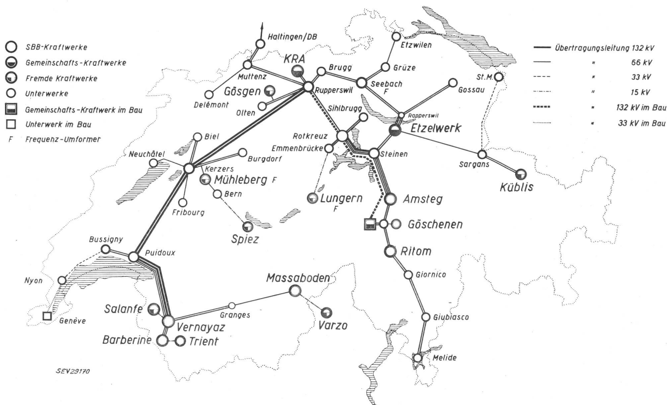
Fig. 1 Kraftwerke, Unterwerke und Übertragungsleitungen der SBB
