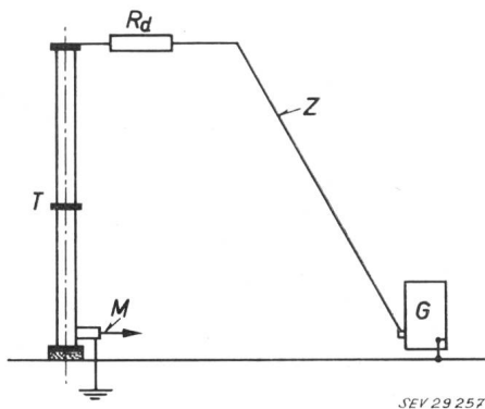
Fig. 21 Eichung der 0,6-MV-Messanordnung mit Rechteckstoss T kapazitiver Spannungsteiler; R_d Dämpfungswiderstand; Z Zuleitung; G Rechteckstossgenerator; M Messkabel
