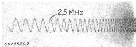
Fig. 26 Eichfrequenz des 5,0- \mu\text{s} -Zeitablaufes Eichfrequenz f = 2,5 \text{ MHz}
