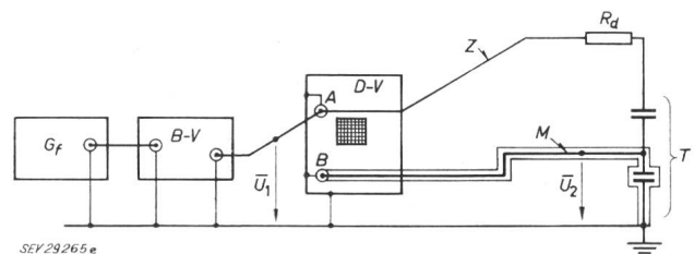
Fig. 29 Prinzipschema der 0,6-MV-Messanordnung für Stoss zur Messung der Phasenverschiebung und des Amplitudenganges G_f Frequenzgenerator; B-V Breitbandverstärker; D-V Differentialverstärker mit Eingängen «A» und «B»; Z Zuleitung; R_d Dämpfungswiderstand; T kapazitiver Spannungsteiler; M Messkabel; U_1 angelegte Wechselspannung; U_2 übertragene Wechselspannung
