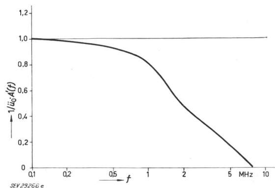
Fig. 30 Amplitudengang der 0,6-MV-Messanordnung \frac{1}{u_0} A'(f) Amplitudengang; f Frequenz
