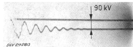
Fig. 24 Rechteckstossantwort der 0,6-MV-Messanordnung ohne Dämpfungswiderstand bei angelegtem 90-kV-Rechteckstoss Zeitablauf 5,0 \mu s (logarithmisch); Resonanzfrequenz f_r = 2,0 MHz
