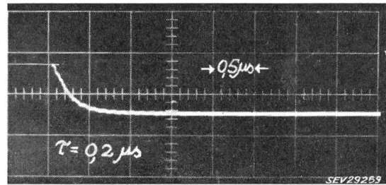
Fig. 23 Niederspannungs-Rechteckstossantwort der 0,6-MV-Messanordnung mit R_d = 400 \Omega Dämpfungswiderstand Zeitablaufgeschwindigkeit 0,5 \mu s/cm; Zeitkonstante der Antwort \tau = 0,2 \mu s
