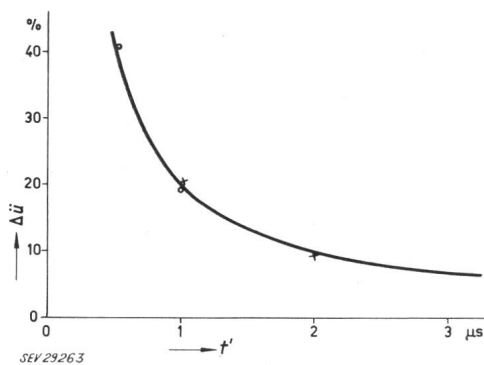
Fig. 27 Übertragungsfehler der 0,6-MV-Messanordnung mit 400 \Omega Dämpfungswiderstand bei Steilstoss \Delta\ddot{u} prozentualer Übertragungsfehler; t' Abschneidezeit; Kurve: Aus der Rechteckstossantwort erhalten; 0, X Messpunkte, welche durch die Frequenzgangmethode — Zerlegung der periodischen Funktionen s_1(t) und s_2(t) — erhalten wurden
