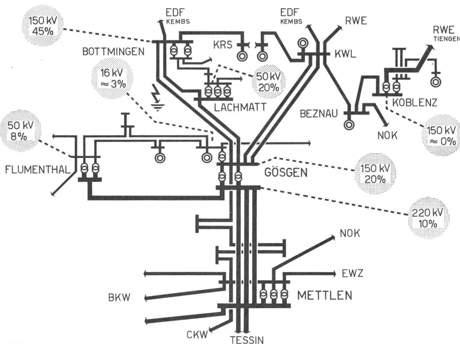
Fig. 8 Spannungsabsenkungen an verschiedenen Netzpunkten während eines Erdkurzschlussversuches auf der 150-kV-Leitung Gösgen–Bottmingen
