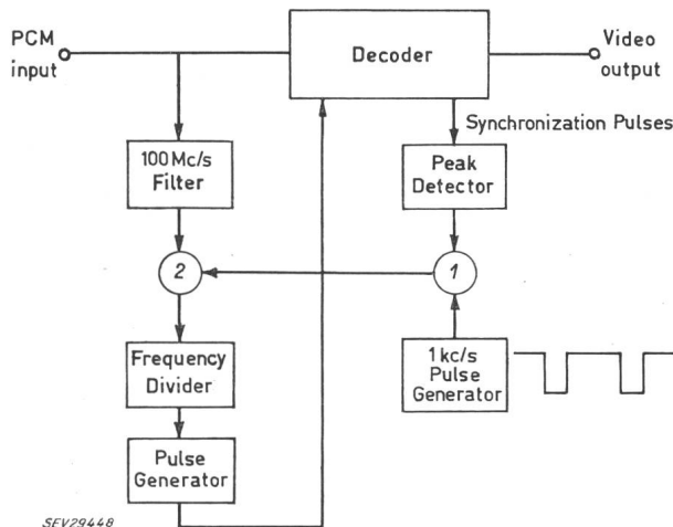
Fig. 15 Synchronizer
