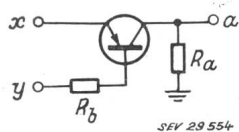
Fig. 2 Sperrgatter für positive Spannungen y ist der Sperreingang. Für negative Spannungen nimmt man einen npn-Transistor
