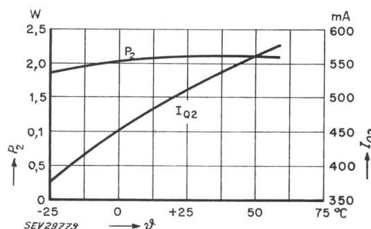
Fig. 3 Kollektor-Ruehstrom des Ausgangstransistors und Ausgangsleistung in Funktion der Umgebungstemperatur \vartheta Umgebungstemperatur ( ^{\circ}C ); P_2 Ausgangsleistung; I_{Q2} Ruhestrom
