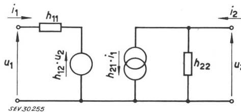
Schéma équivalent à un transistor donné par ses paramètres h Indications voir fig. 1
