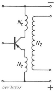
Fig. 5 Schéma de principe du montage «split-load» N_e Enroulement de collecteur; N_e Enroulement d'émetteur; N_2 Enroulement secondaire
