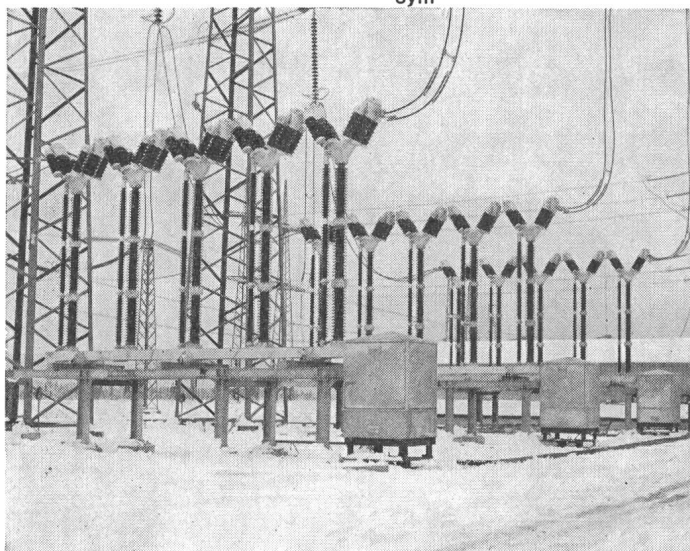
Ölarmes Leistungsschalter Typ HPF 516 in Kilforsen, Schweden
