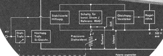
Vereinfachtes Prinzipschema
