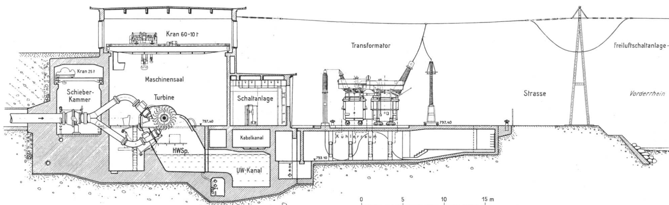
Fig. 5 Querschnitt durch das Maschinenhaus des Kraftwerkes Tavanasa
