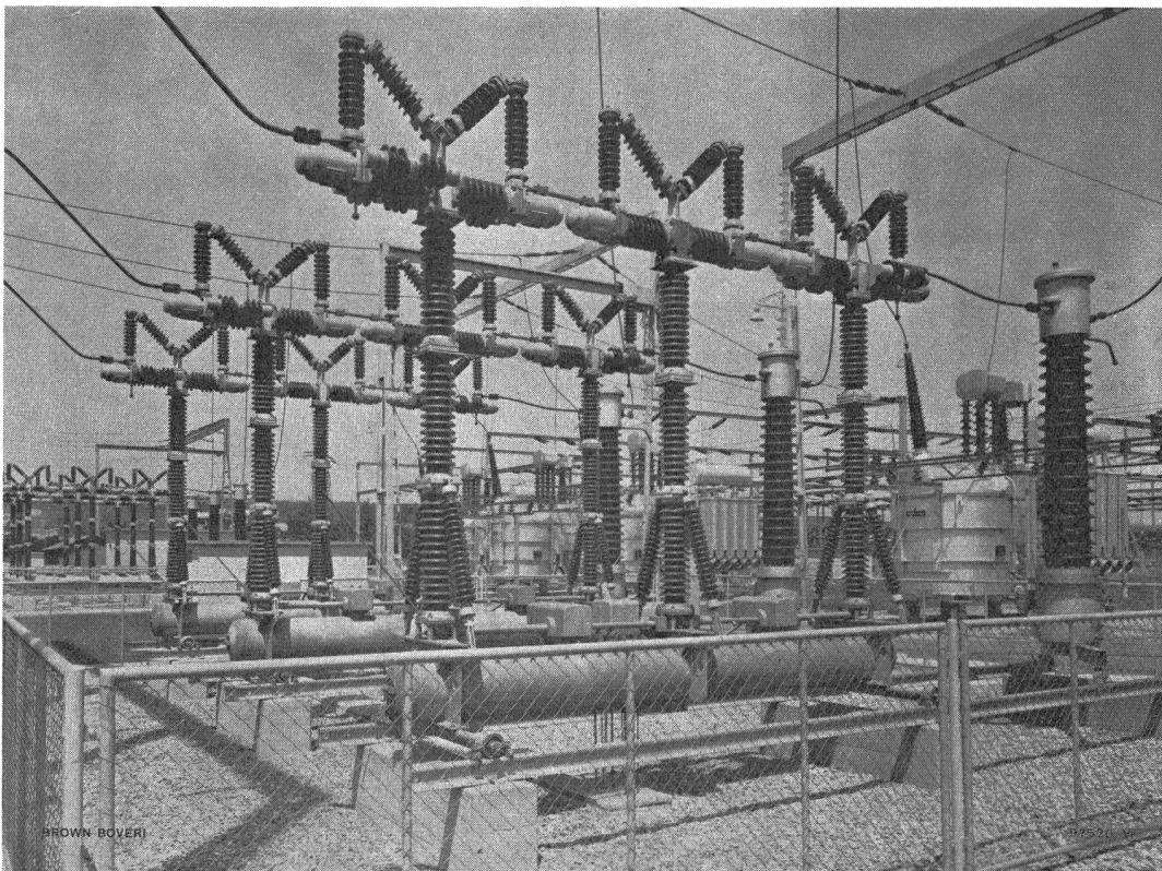
Teil der 220-kV-Freiluftanlage Laufenburg/Schweiz mit 220-kV-Druckluftschneckschaltern. Im Hintergrund eine einphasige Auto-Stufentransformatorgruppe für 125 MVA, 220/150kV.
