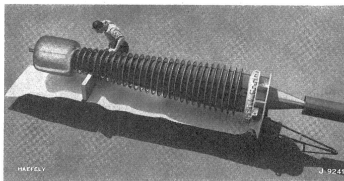
Transformator-Durchführung 420 kV
