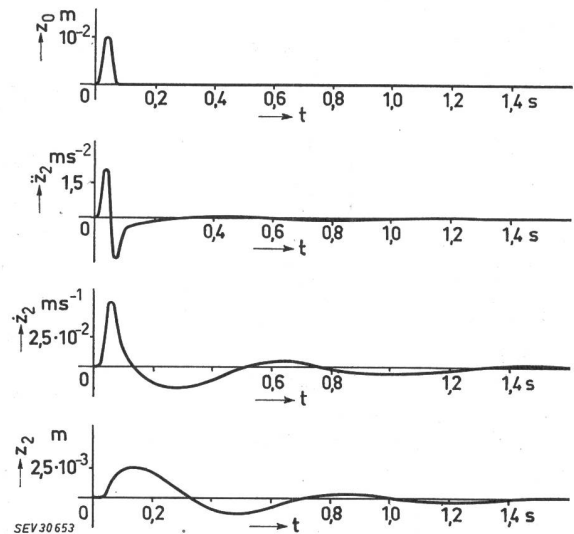
Fig. 8 Mit dem Analogierechnergerät erhaltene Lösungskurven Von oben nach unten sind dargestellt: Verlauf der Unebenheit, Beschleunigung, Geschwindigkeit und Auslenkung der Masse m
