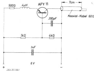
Fig. 7 Oszillator 500 MHz
