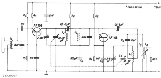
Fig. 8 UKW-Tuner 86...102 MHz
