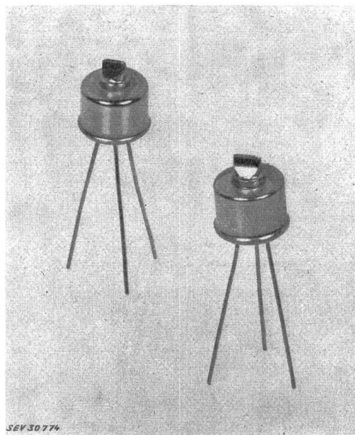
Fig. 1 Mesa-Transistoren
