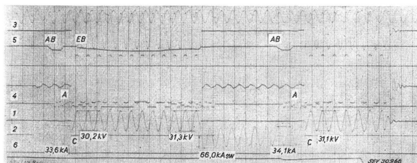
Fig. 13 Oszillogramm eines O-CO-Kurzschlusses bei erhöhter Leistung
