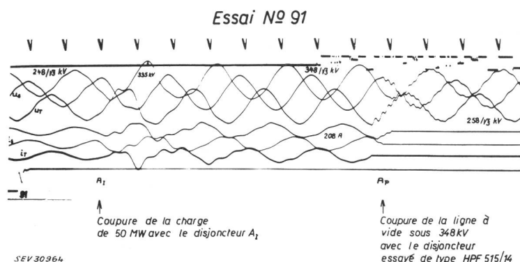
Fig. 11 Oszillogramm einer 220-kV-Leitungsabschaltung nach Lastabwurf bei 330 kV
