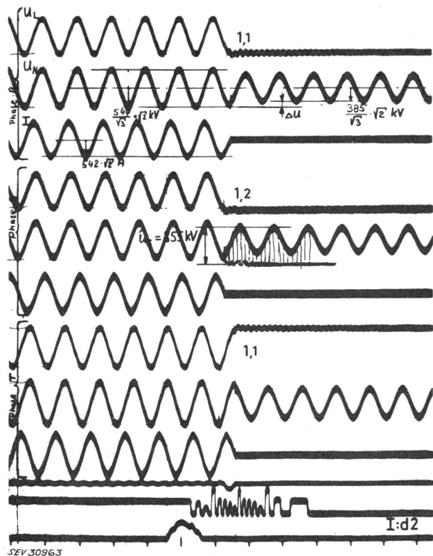
Oszillogramm der Abschaltung einer leerlaufenden 420-kV-Leitung unter überhöhter Spannung (540 kV, Schweden)
