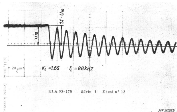
Fig. 12 Oszillogramm des leitungsseitigen Spannungsanstieges beim Abstandskurzschluss Aufgenommen in Fontenay (Frankreich)
