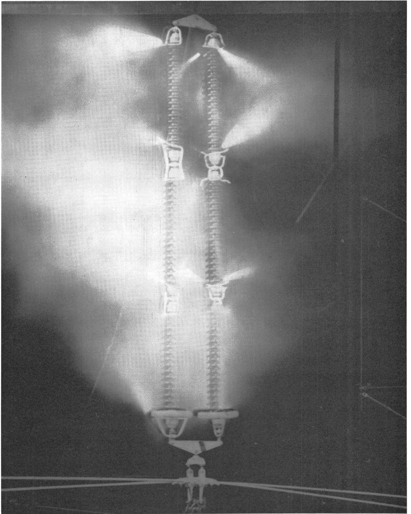
Hochstromversuch ausgeführt mit NORDEN LANGSTABISOLATOREN bei KEMA, Arnhem, Holland. Stromstärke 26.000 Amp. während 0,30 Sek.
