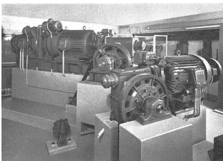
Neuzeitliche Maschinengruppe einer Doppelaufzugsanlage mit fremdbelüfteten, mehrtourigen, gekapselten Antriebsmotoren.
