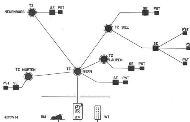
Fig. 15 Blockschema der Fernmeldeanlagen des Bureaus für Wassernutzung, Bern P 'ST Pegelstation; SE Sender; EP Empfänger; TZ Telephonzentrale; RM Registriermaschine; WT Wahltableau; U Weckeruhr; EK elektrischer Kalender
