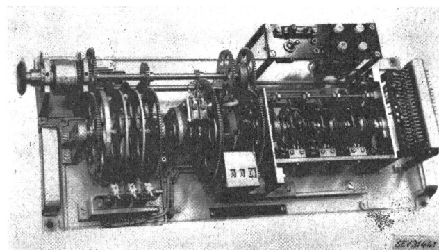
Fig. 22 Umrechnungseinheit mit mehrstufigem Magnetspeicher und Summier-Dekadenkontaktwerk
