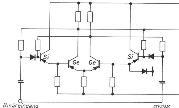
Fig. 10 Untersetzer
