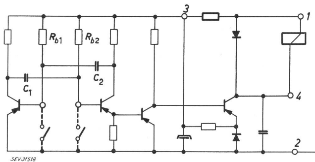
Fig. 8 Impulsgenerator
