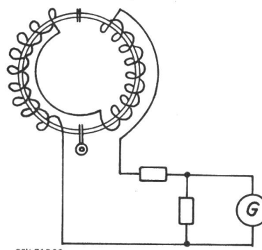
Fig. 2 Solenoid mit Galvanometer
