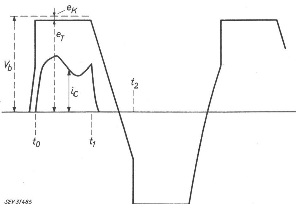
Fig. 9 Verlauf der Transformatorspannung und des daraus folgenden Kollektorstromes
