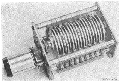
Fig. 1 Programmsteuerung Typ 212
