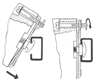
Fig. 2 «Isobloc»-Sicherungselement
