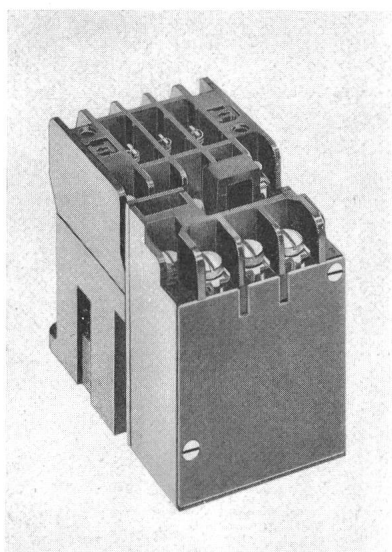
Fig. 2 Schütz mit Thermoblock für 16 A, 500 V
