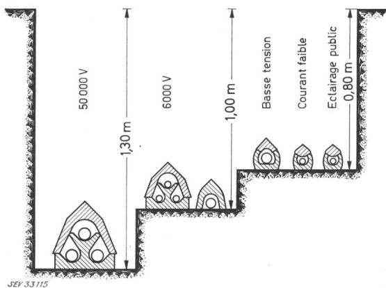
Fig. 11 Croquis montrant la disposition des câbles, sous caniveaux type Rütchi, dans le sous-sol lausannois
