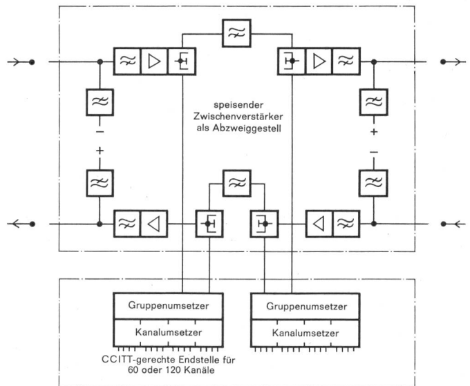
SEV 33329 Fig. 8 Übersichtsstromlauf einer Abzweigstelle mit Wiederbelegung
