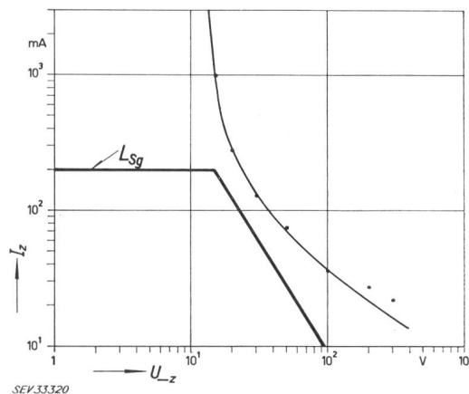
Fig. 12 Zündung von Schwefelkohlenstoff-Luft-Gemischen mit Ohmschen Stromkreisen (Induktivität < 100 \mu\text{H} ) Schwefelkohlenstoff 60 \mu\text{l} Weitere Bezeichnungen siehe Fig. 6
