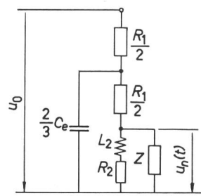
Fig. 7 Ersatzschaltbild eines inhomogenen Ohmschen Spannungsteilers L_2 Zusatzinduktivität des Niederspannungsteiles; Z Ersatzwiderstand des Messkabels Weitere Bezeichnungen siehe Fig. 5 und 6
