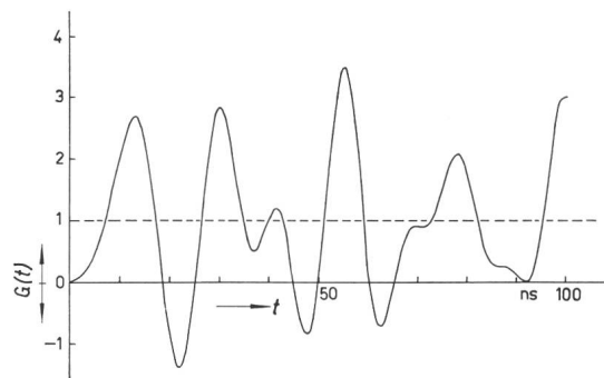
Fig. 8 Übergangsfunktion eines rein kapazitiven Spannungsteilers G(t) Übergangsfunktion; t Zeit C = 150 pF; C_e = 40 pF; C_p = 1 pF; L = 2,5 \mu H; R = 20 \Omega Bedeutung dieser Grössen siehe Fig. 9
