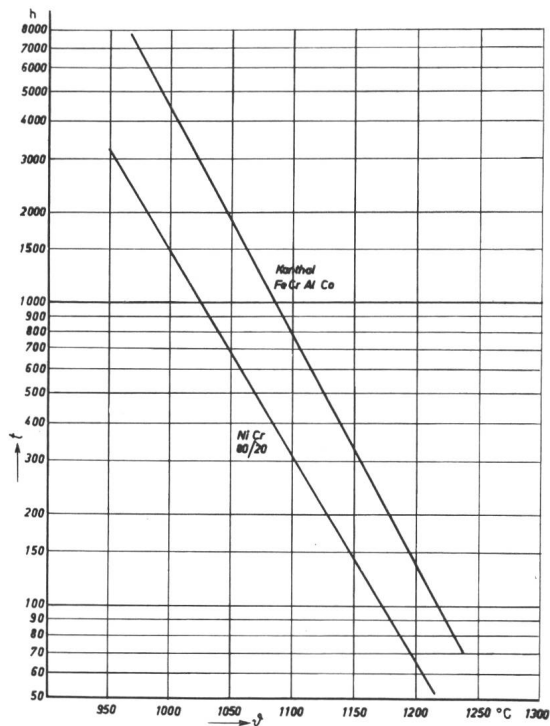
Fig. 2 Lebensdauer t in Abhängigkeit von der Temperatur \theta
