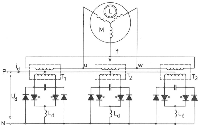
Fig. 61 Dreiphasiger selbstgeführter Wechselrichter für Drehstrommotorspeisung P, N Gleichspannungsnetz; T 1 , T 2 , T 3 Transformatoren; M Statorwicklung des Asynchronmotors; L Läufer; f Statorfrequenz; U d Gleichspannung; i a Gleichstrom; L d Glättungsinduktivität
