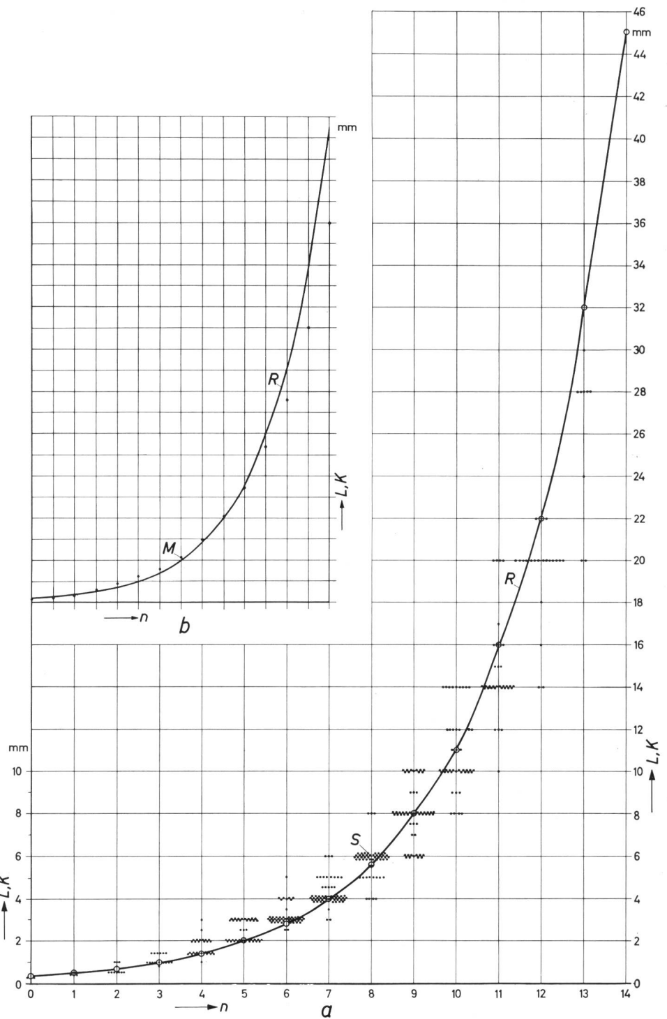
Fig. 4 Normstrecken der Tabelle III in Funktion des Bewertungsexponenten und Vergleich mit den Streuwerten ( a ) und deren Mittelwert ( b ) (s. Tabelle V) L Luftstrecke; K Kriechstrecke; M Mittelwert der Streuwerte; S Streuwerte; R Normstreckenkurve; n Bewertungsexponent
