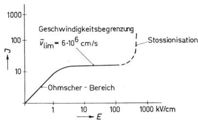
Fig. 8 Strom-Spannungscharakteristik eines Siliziumkristalles
