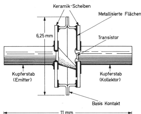
Fig. 22 Aufbau eines Koaxialtransistors (Bild Texas Instr.)
