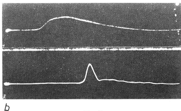
Fig. 10 Impulsverkürzung
