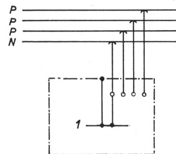
Fig. 12 Ausführung unzulässig
