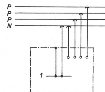
Fig. 13 Ausführung bei Nullung nach Schema III
